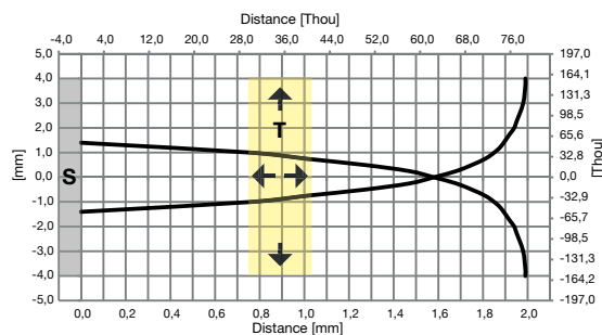
Fig. 2 Flush, 2mm
